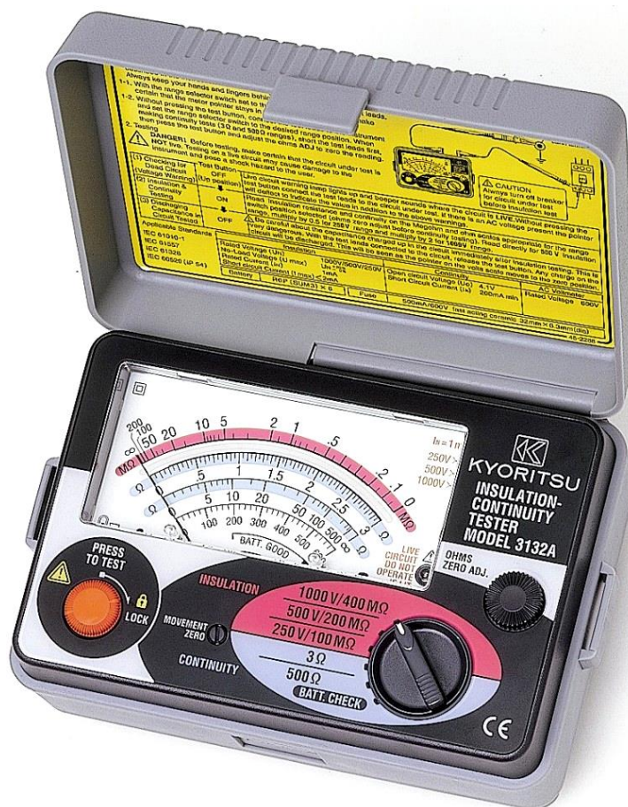
Рисунок 15 – Общий вид мегаомметров KEW 3132A
